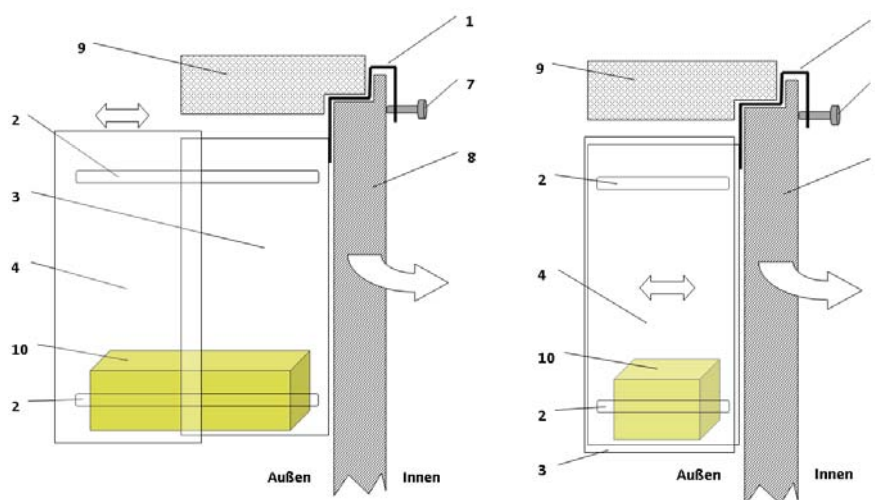
Huckepack Paket-Box Seitenansicht ausgefahren (links); eingefahren (rechts)
